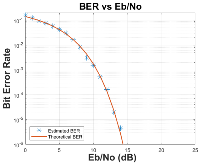
Fig. 13. BER vs. EbNo. (dB)
